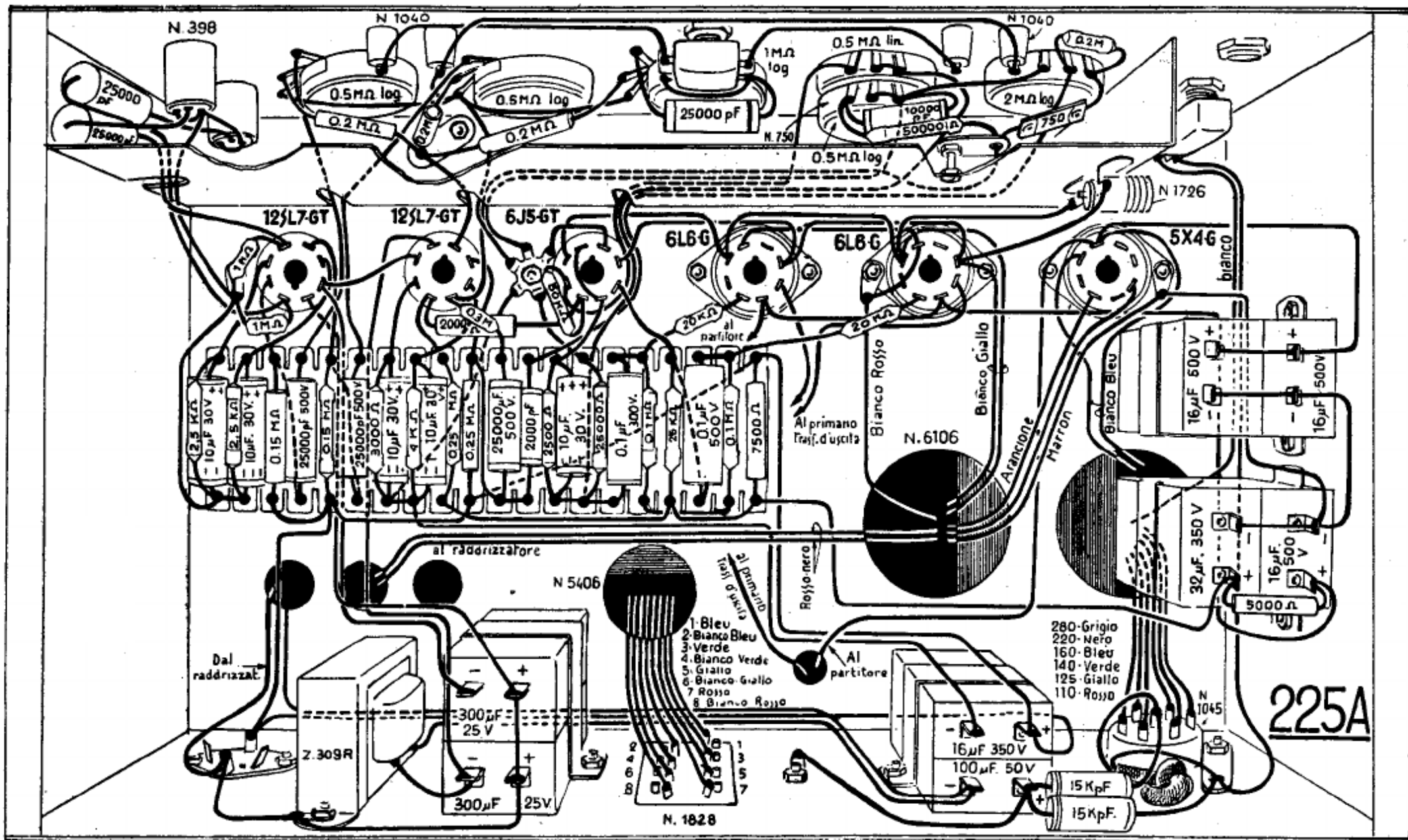
Lo schema costruttivo del G-225/A.
